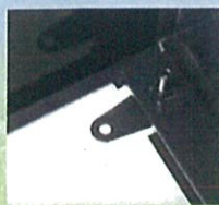
水勾配対応アジャスター (30mm までの段差に対応)
